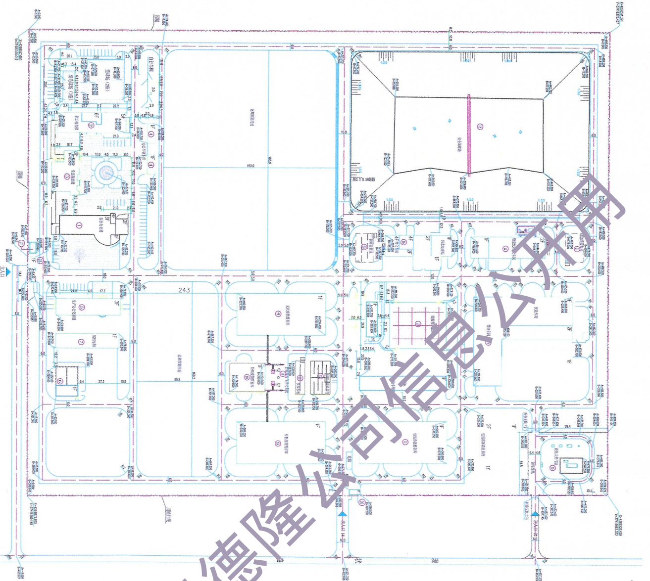
图2.2-2 项目平面布置图
